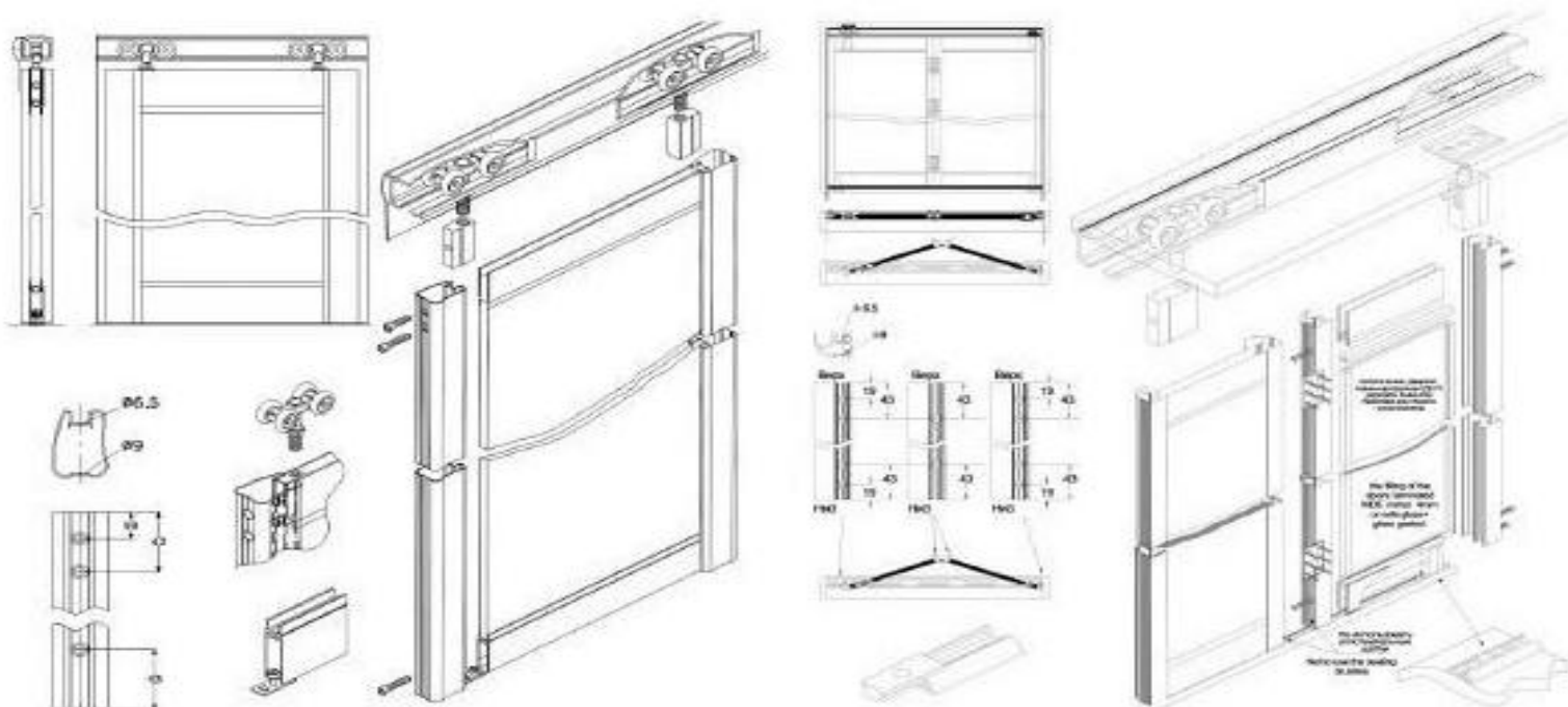
Комплект для подвесной системы
